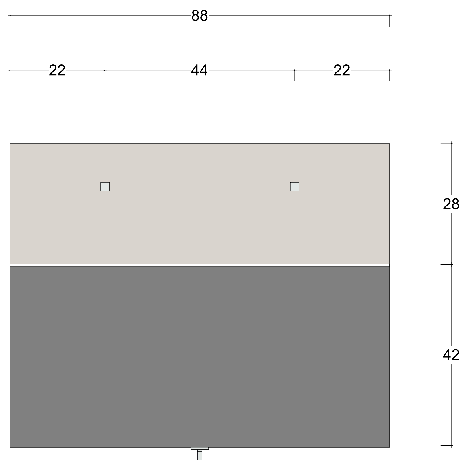
T LOCKERS - GA PLAN Scale: 1:5
