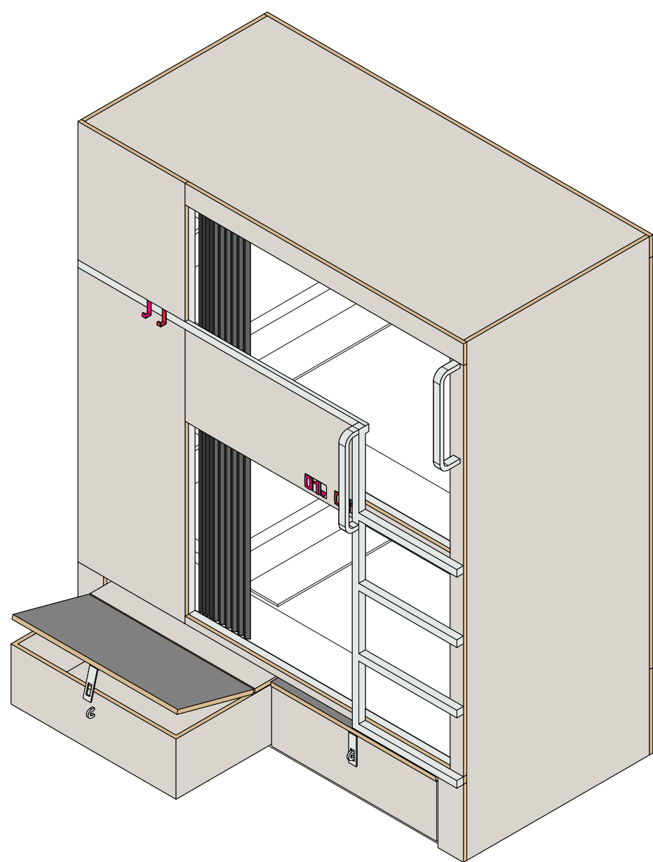
BUNKBED 2-A QTY: 26
